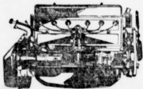
Le nouvel engin six cylindres du Chevrolet, complètement recouvert, soupapes-en-tête, haute compression, tête non-détonnante, 194 pouces cubes pour le déplacement du piston et développant 45 c.v. à petits vitesses du moteur.
