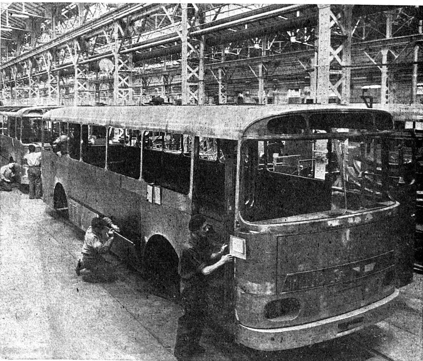
Montage d'autocars (de 14 à 60 places) — d'autobus (de 45 à 180 places) et de trolleybus (de 85 à 180 places).
