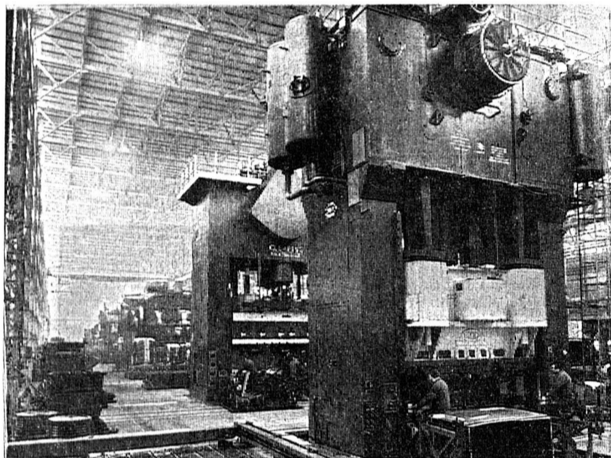
Presses de 900 et 1200 tonnes de puissance dans l'atelier d'emboutissage.
