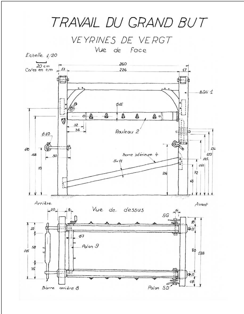
Fig. 5. Travail du Grand But, relevé, vue de face et vue de dessus.
