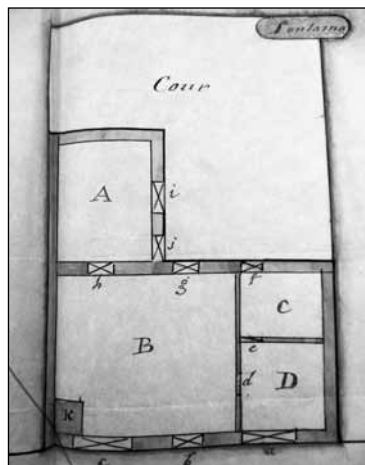
Fig. 7. Plan détaillé des locaux de la fabrique projetée Rouchaud & Girard (photo Catherine Charles). a, b, c : portails et porte d'entrée du rez-de-chaussée donnant sur la rue de circulation. d, e, f, g, h, i, j : portes de séparation et de communication, croisées. k : réservoir d'eau. A : local de la chaudière. B : local destinés aux foulons (fabrication de la cloche). C : bureau de l'usine. D : atelier d'appropriage ( finition du chapeau). Au-dessus des points B, C, D se trouve le grenier.
