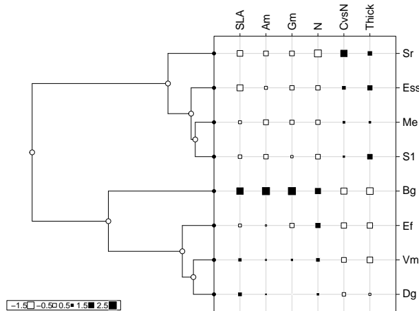
FIG. 7.10 : Présentation de l'arbre phylogénétique avec la contribution de chacune des variables.
