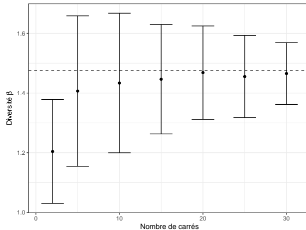
FIG. 12.1 : Estimation de la diversité \beta entre carrés de BCI. La diversité est calculée à partir du nombre de carrés en abscisse, de 2 à 30, tirés aléatoirement. La valeur en ordonnée est la diversité d'ordre 2 moyenne sur 100 tirages, les barres représentent l'écart-type. Aux erreurs d'estimation près et dès 5 carrés (nécessaires pour représenter l'ensemble du dispositif), la valeur de la diversité \beta ne dépend pas du nombre de carrés. La ligne horizontale représente la diversité \beta entre tous les carrés.
