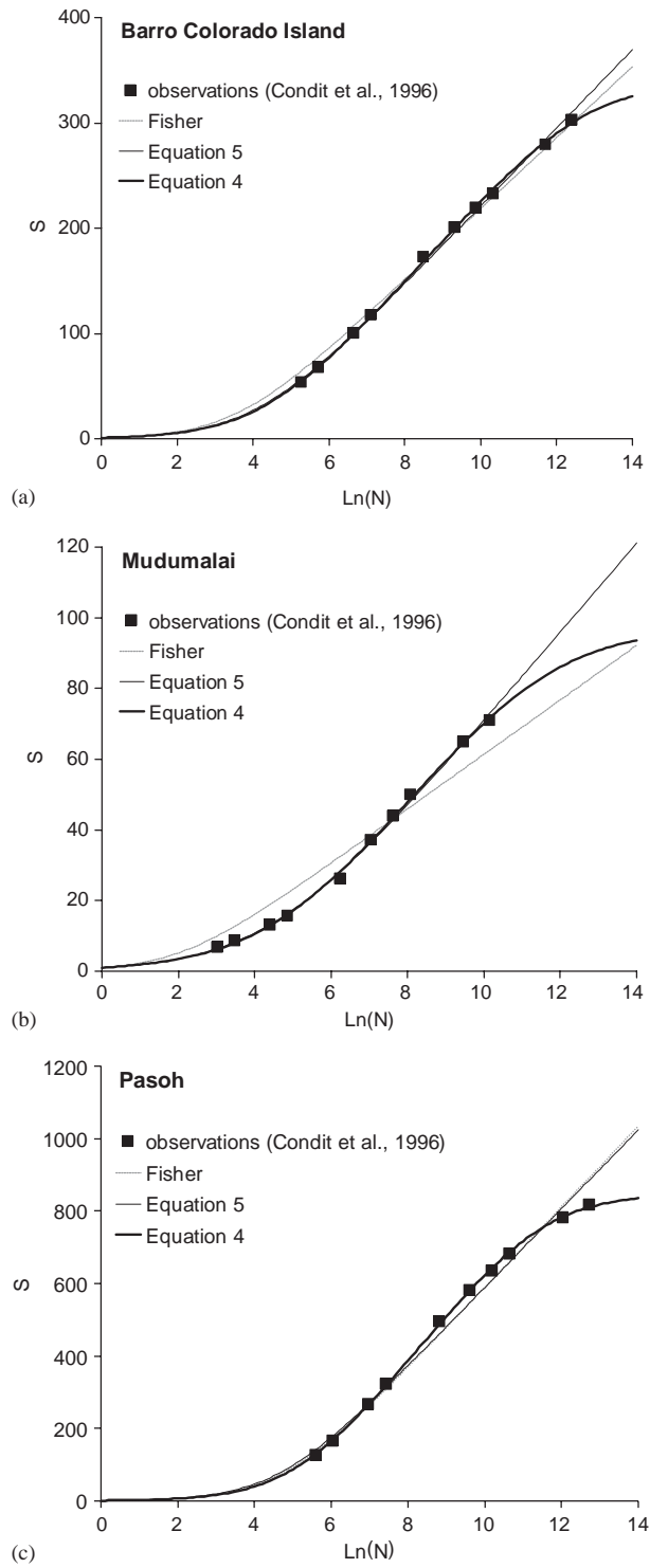
FIG. 20.4 : Comparaison entre le modèle de Fisher et le modèle étendu dans trois parcelles forestières connues. Les modèles sont ajustés aux données. Les courbes légendées Equation 4 correspondent au modèle de Fisher étendu par Schulte, alors que l' Equation 5 est le modèle intermédiaire, supposant le nombre total d'espèces infini.
