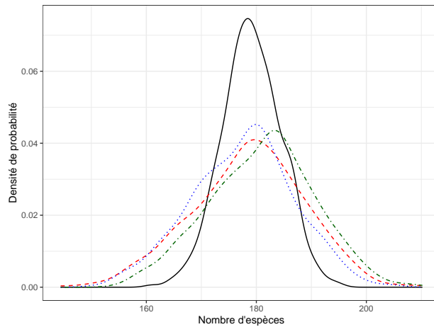
FIG. 21.4 : Distribution de la richesse obtenue par extrapolation à 1800 individus de 500 inventaires de 1000 individus selon les méthodes de Shen et al. (pointillés alternés vert), Béguinot (tirets rouges) ou Chao, Gotelli et al. (pointillés bleu). La distribution de la richesse de 500 inventaires de même taille est représentée par la courbe noire.
