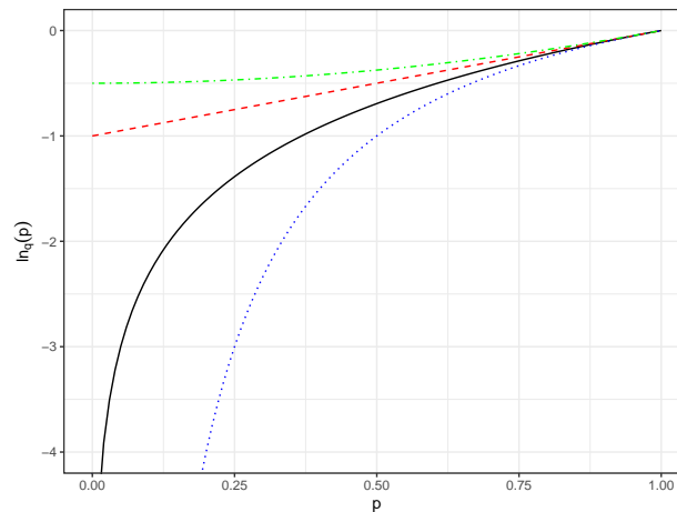
FIG. 4.4 : Valeur du logarithme d'ordre q de probabilités entre 0 et 1 pour différentes valeurs de q : q = 0 (pointillés longs rouges), la courbe est une droite ; q = 1 (trait plein) : logarithme naturel ; q = 2 (pointillés courts bleus) : la courbe a la même forme que le logarithme naturel pour les valeurs positives de q ; q = -1 (pointillés alternés verts) : la courbe est convexe pour les valeurs négatives de q .
