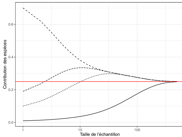
FIG. 7.3 : Contribution des espèces à l'indice de Hurlbert. Les contributions de 4 espèces d'une communauté à l'indice sont représentées en fonction de la taille de l'échantillon n . Les fréquences des espèces sont lisibles pour n = 1 : une espèce fréquente (probabilité égale à 0,7, supérieure à 1/S ), deux espèces peu fréquentes (0,19 et 0,1), et une espèce rare (0,01). Quand n est assez grand, toutes les contributions tendent vers 1/S = 1/4 (ligne horizontale).
