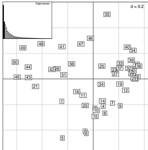
FIG. 11.8 : PCoA appliquée à la distance de corde des 50 carrés de BCI pour visualiser la diversité \beta .
