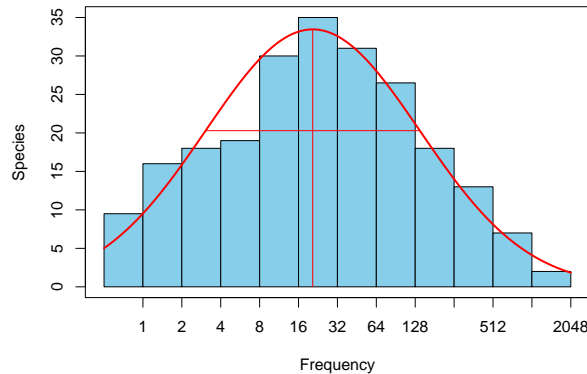
FIG. 3.5 : Ajustement du modèle de Preston aux données de BCI.
