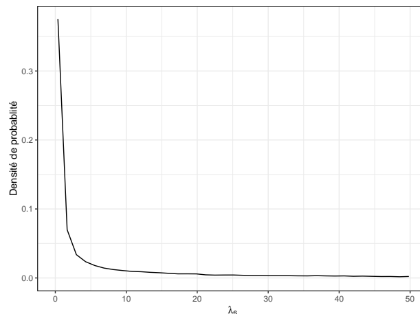
FIG. 20.1 : Densité de probabilité d'une loi gamma de paramètres 0, 2 et 100. Seules les valeurs inférieures à 50 sont affichées.
