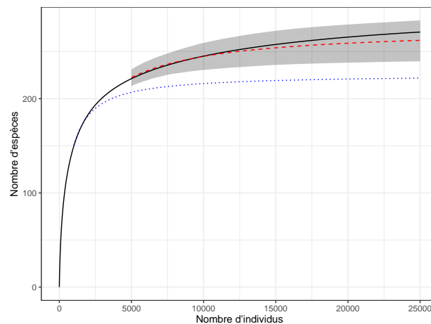
FIG. 21.5 : Extrapolation de 500 inventaires de 5000 individus (valeurs moyenne en tireté rouge et enveloppe de confiance à 95% en gris) superposée à la SAC réelle d'une communauté log-normale de 300 espèces. L'extrapolation (en pointillés bleu) d'un inventaire limité à 1000 individus est sévèrement sous-estimée.
