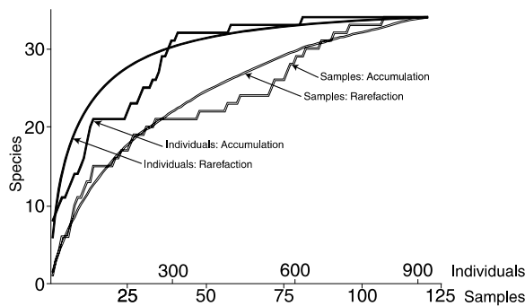
FIG. 21.1 : Courbes d'accumulation et de raréfaction, obtenues par inventaires individuels ou groupés ( samples ). Les courbes de raréfaction permettent de lisser les courbes d'accumulation. Les courbes obtenues par inventaire groupé sont en général en dessous des courbes individuelles à cause de l'agrégation spatiale.
