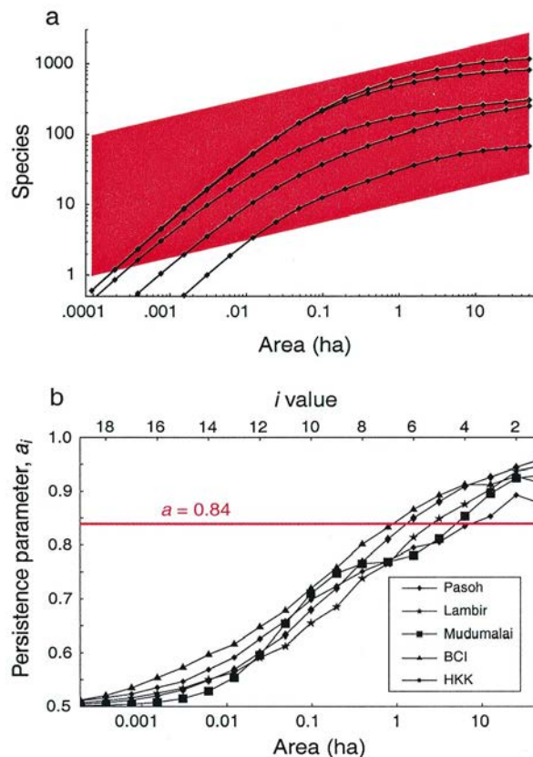
FIG. 22.3 : Courbes aire-espèces (a) et paramètre de persistance en fonction de la surface (b) dans 5 forêts tropicales. Le modèle d'Arrhenius est représentée par le parallélogramme sur la figure a, pour une gamme de valeurs de la constante. Elle implique que la relation aire-espèces représentée en logarithmes soit une droite, dont la position dépend de la constante, ce qui n'est visiblement pas le cas.
