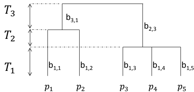
FIG. 7.4 : Arbre phylogénétique ou fonctionnel hypothétique.
