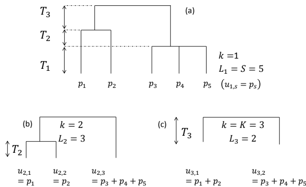
FIG. 7.7 : Arbre phylogénétique ou fonctionnel hypothétique. (a) Arbre complet. 5 espèces sont présentes ( S = 5 ). Une période de l'arbre est définie entre deux noeuds successifs : l'arbre contient K = 3 périodes. Les hauteurs des périodes sont notées T_k . À chaque période correspond un arbre plus simple : (b) pour la période 2, (c) pour la période 3 dans lequel les espèces originales sont regroupées. Le nombre de feuilles de ces arbres est noté L_k . Les probabilités pour un individu d'appartenir à une feuille sont notées u_{k,l} .
