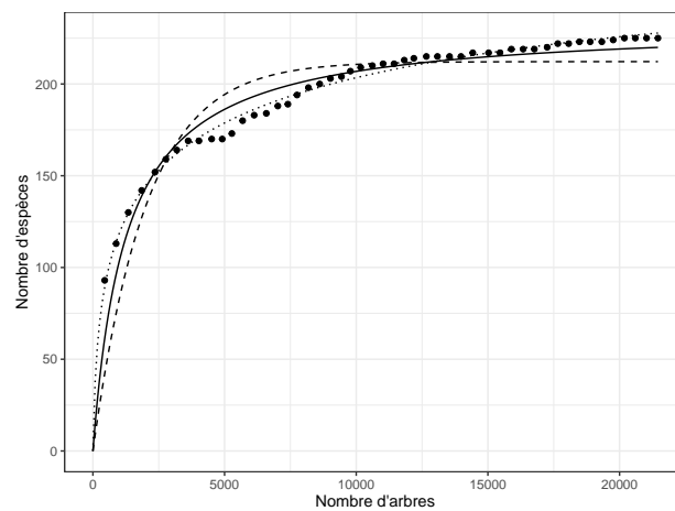
FIG. 3.7 : Ajustement des modèle de Michaelis-Menten (trait plein) et de de Soberón et Llorente (pointillés longs : modèle exponentiel négatif; pointillés courts : modèle à trois paramètres) aux données de BCI. Les cercles représentent le nombre d'espèces cumulées en fonction du nombre d'arbres. Le modèle exponentiel négatif (Holdridge) sous-estime la richesse, plus que celui de Michaelis-Menten (Clench). Le modèle à trois paramètres s'ajuste mieux aux données, mais il surestime probablement la richesse.
