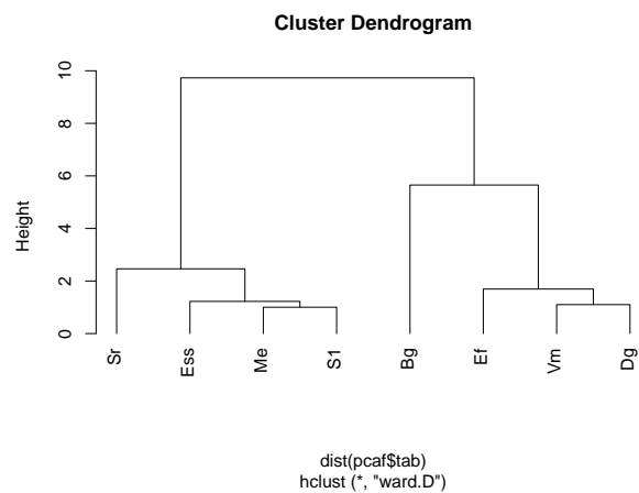
FIG. 7.9 : Arbre phylogénétique issu de la classification automatique.
