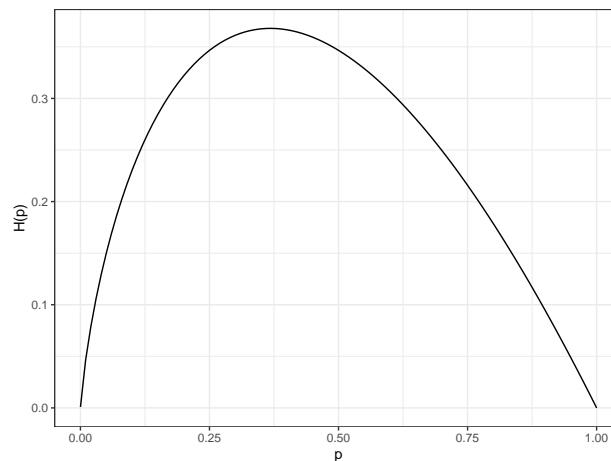
FIG. 3.9 : Courbe de x \ln x entre 0 et 1.
