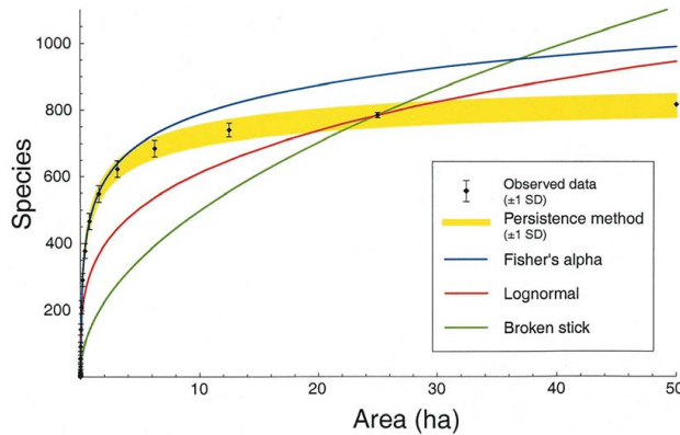
FIG. 22.4 : Performance du modèle de Plotkin face à des distributions théoriques : SAD log-normales, modèles de Fisher et Broken Stick de MacArthur. La courbe représente le nombre d'espèces rencontrées à Pasoh sur des surfaces de 0 à 50 ha. Les données observées sont des tirages aléatoires d'échantillons de la surface souhaitée. L'écart-type est représenté (l'intervalle de fluctuation à 95% est de l'ordre de 2 écart-types). Les valeurs issues du modèle ont été obtenues par un paramétrage de k et z sur 25 ha, supposé valide également sur les autres forêts. Le paramétrage de c est obtenu par un échantillon d'un hectare, répété 1000 fois pour obtenir un intervalle de confiance. L'intervalle de fluctuation à 95% est ici encore de l'ordre de deux écart-types.
