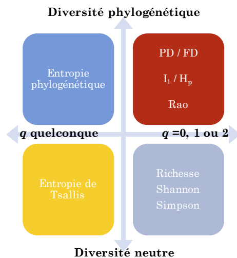
FIG. 24.1 : Généralisation des mesures classiques de diversité. La figure présente les mesures d'entropie, qui peuvent toutes être transformées en mesures de diversité au sens strict. Toutes ces entropies sont des cas particuliers de l'entropie de Ricotta et Szeidl, qui peut être transformée en diversité de Leinster et Cobbold.
