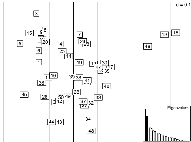
FIG. 11.3 : Représentation des 50 carrés de BCI dans une analyse en coordonnées principale fondée sur les distances de Jaccard.
