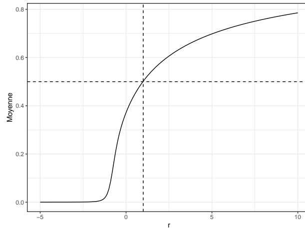
FIG. 9.1 : Moyenne généralisée d'ordre r (en abscisse) d'une distribution uniforme de 10000 valeurs tirées entre 0 et 1. La moyenne arithmétique 0,5 est obtenue pour r = 1 . La moyenne généralisée tend vers la plus petite valeur (près de 0) quand r \rightarrow -\infty , et vers la plus grande valeur (près de 1) quand r \rightarrow +\infty .
