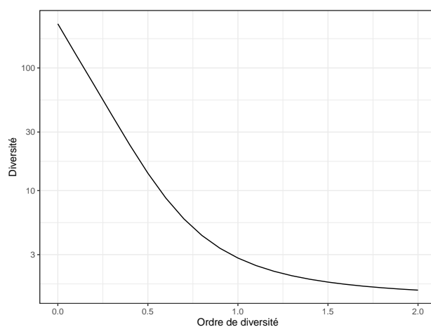
FIG. 9.6 : Profil de diversité des valeurs propres de la méta-communauté Paracou618.
