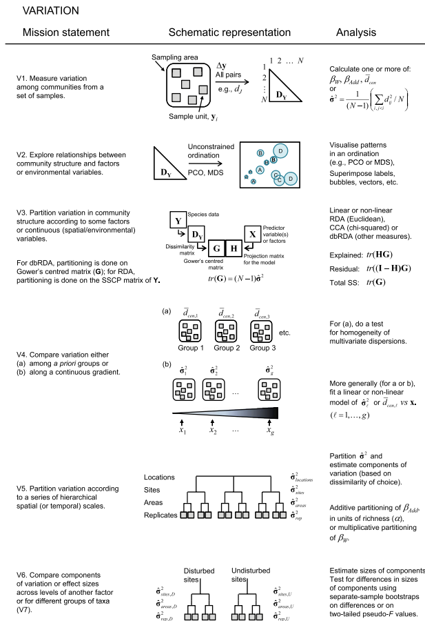
FIG. 10.2 : Diversité \beta liée à la variation de la composition spécifique. \beta_W est le rapport entre la diversité \gamma et la diversité \alpha , \beta_{Add} leur différence. d_{ij} est la dissimilarité entre les communautés i et j . \hat{\sigma}^2 est la variance de cette dissimilarité, \bar{d} sa moyenne. Si d est une distance euclidienne, \bar{d}_{cen} est la distance moyenne des communautés à leur centre de gravité.
