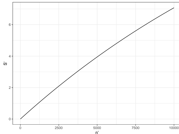
FIG. 3.4 : Nombre de nouvelles espèces découvertes en fonction de l'effort d'échantillonnage supplémentaire (données de BCI). Seulement 7 nouvelles espèces seront observées en échantillonnant 10000 arbres supplémentaires (environ 25 ha en plus des 50 ha de la parcelle qui contiennent 225 espèces).
