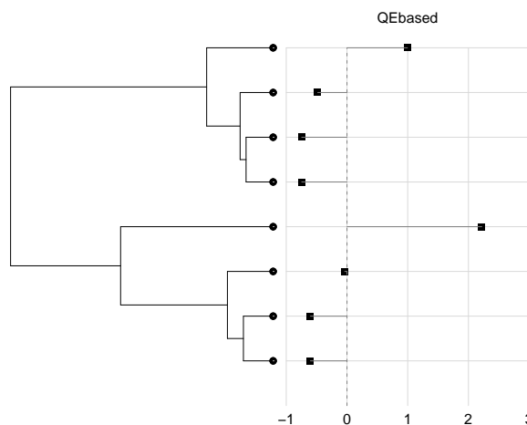
FIG. 7.11 : Originalité des espèces.
