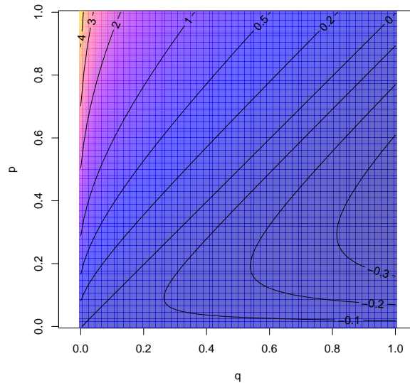
FIG. 4.3 : Valeur de q \ln(q/p) en fonction de p et q . La divergence de Kullback-Leibler est la somme de cette valeur pour toutes les espèces
