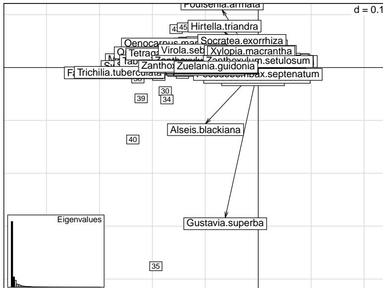
FIG. 11.5 : Représentation des deux premiers axes factoriels de l’ACP des 50 carrés de BCI. Les données sont les probabilités des espèces, ni centrées ni réduites pour l’ACP. Les carrés sont représentés avec les espèces. Les carrés 35 et 40 ont une diversité faible et sont associés aux espèces Gustavia superba et Alseis blackiana .
