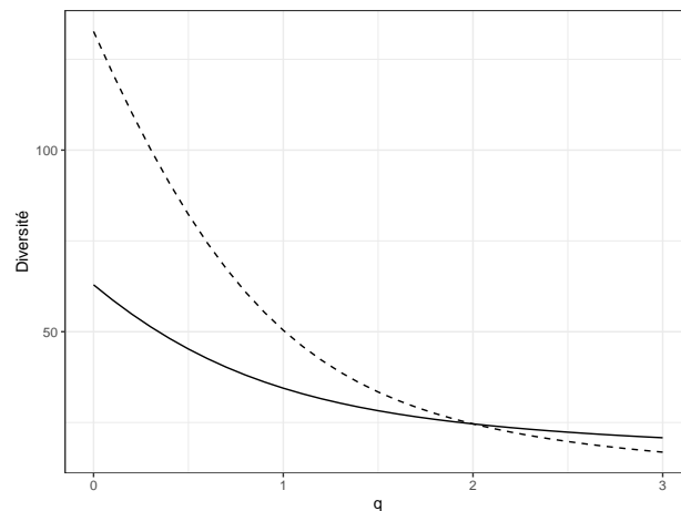
FIG. 9.7 : Diversité phylogénétique (l'arbre est une taxonomie) d'ordre q de deux hectares de forêt de Paracou : qD^{\mathbf{Z}} (trait plein) et q\hat{D}(T) (pointillé).
