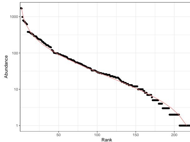
FIG. 2.3 : Diagramme rang-abondance (diagramme de Whittaker) des arbres du dispositif de Barro Colorado Island. Les points sont les données : en abscisse : le rang de l'espèce, à partir de la plus abondante ; en ordonnée : l'abondance de l'espèce. La courbe est l'ajustement d'une distribution log-normale.
