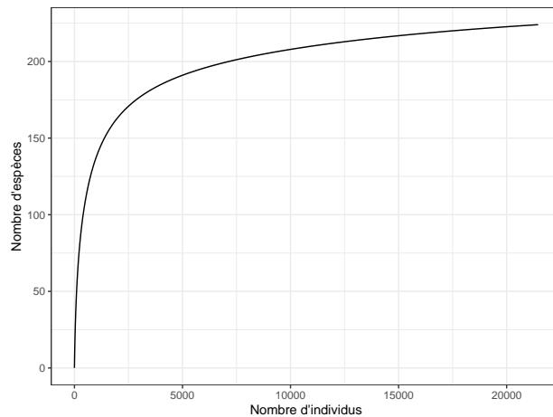
FIG. 21.3 : Courbe d'accumulation des espèces d'arbres de Barro Colorado Island. Somme des entropies de Simpson généralisées.
