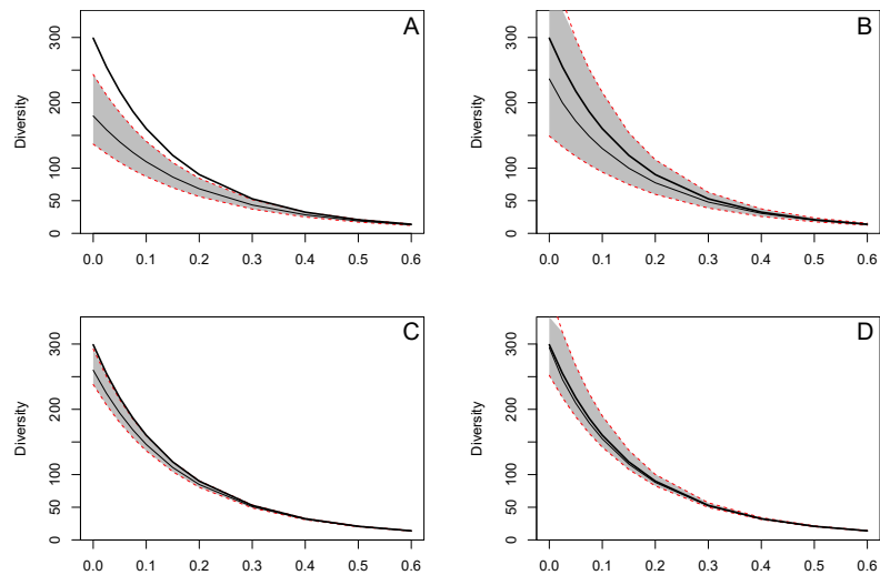
FIG. 4.7 : Estimation de la diversité d'une communauté log-normale de 300 espèces. Un inventaire de 500 (en bas) ou 5000 (en haut) individus est répété 1000 fois et la diversité estimée à chaque fois par l'estimateur de Chao-Wang-Jost (à gauche) ou l'estimateur révélé (à droite). La courbe noire en gras représente la vraie diversité de la communauté. La courbe maigre est la moyenne de l'estimation, l'enveloppe grise limitée par les pointillés rouges contient 95% des valeurs simulées. A : 5000 individus, estimateur de Chao-Wang-Jost. B : 5000 individus, estimateur révélé. C : 500 individus, estimateur de Chao-Wang-Jost. D : 500 individus, estimateur révélé.
