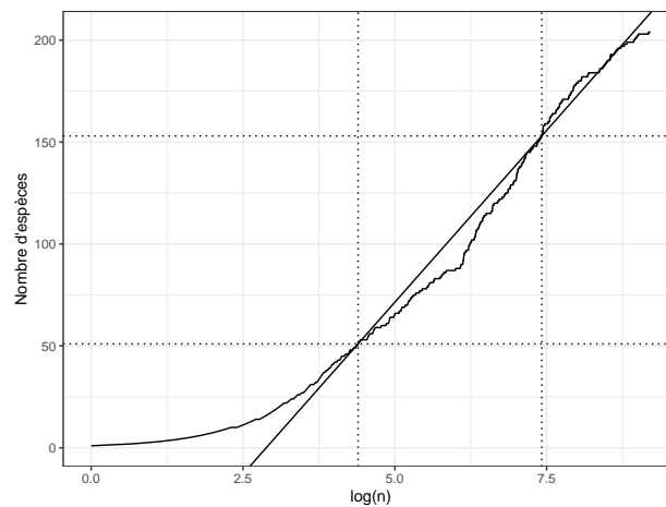
FIG. 20.5 : SAC d'un inventaire simulé de 10000 arbres de BCI. Le nombre d'espèces cumulé est tracé en fonction du logarithme du nombre d'individus échantillonnés. Q est la pente de la droite passant par les points de la courbe correspondant aux premier et troisième quartiles du nombre d'espèces.
