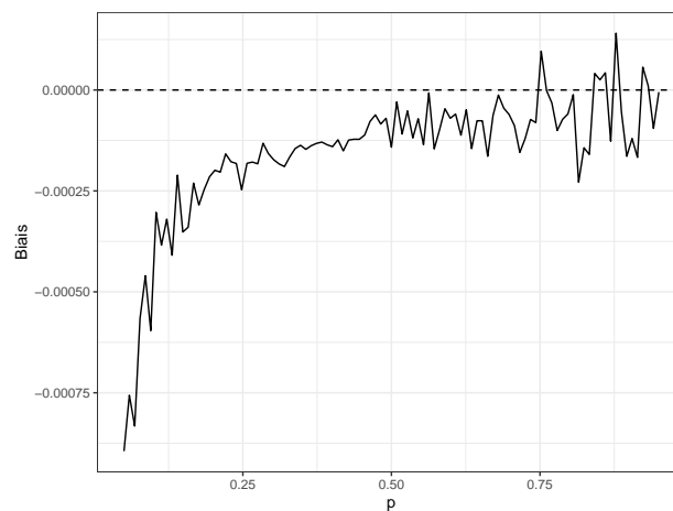
FIG. 3.10 : Biais de \hat{p}_s \ln \hat{p}_s entre 0 et 1.
