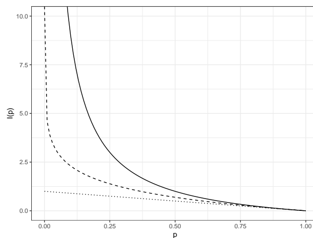
FIG. 4.1 : Fonctions d'information utilisées dans le nombre d'espèces (trait plein), l'indice de Shannon (pointillés longs) et l'indice de Simpson (pointillés). L'information apportée par l'observation d'espèces rares décroît du nombre d'espèces à l'indice de Simpson.
