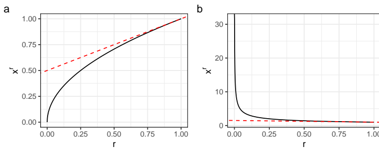
FIG. 9.2 : Approximation de (\mathbf{Zp})_s^{q-1} par son développement limité au premier ordre pour (a) q = 1.5 ( r = q - 1 ) et (b) q = 0.5
