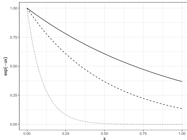
FIG. 9.3 : Transformation des distances (en abscisse) en similarités (en ordonnées) selon la valeur de u . Trait plein : u = 1 ; pointillés longs : u = 2 ; pointillés : u = 10 . Plus u est grand, plus les similarités sont tassées vers 0.
