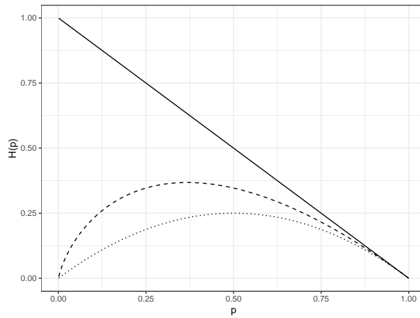
FIG. 4.2 : Valeur de p_s I(p_s) dans le nombre d'espèces (trait plein), l'indice de Shannon (pointillés longs) et l'indice de Simpson (pointillés). Les espèces rares contribuent peu, sauf pour le nombre d'espèces.
