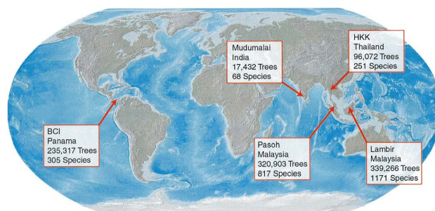
FIG. 22.2 : Les cinq dispositifs de Plotkin et al. Chaque dispositif mesure 50 ha et toutes les tiges de diamètre supérieur à 1 cm sont cartographiées et déterminées.
