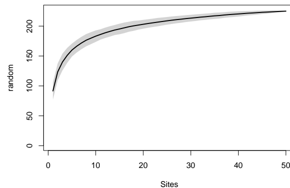
FIG. 21.2 : Courbe d'accumulation des espèces d'arbres de Barro Colorado Island. Calcul par specaccum : accumulation des 50 carrés avec permutations.
