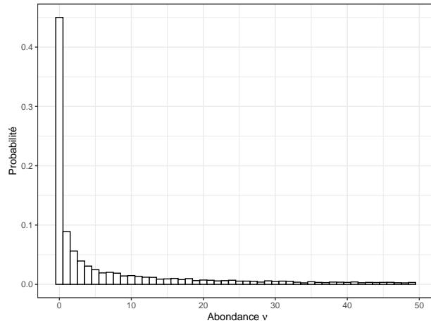
FIG. 20.2 : Réalisation d'une loi gamma de paramètres 0, 2 et 100. L'histogramme représente la proportion (qui estime la probabilité) des valeurs inférieures à 50. Les espèces d'abondance nulle ne sont pas observées dans l'échantillon.
