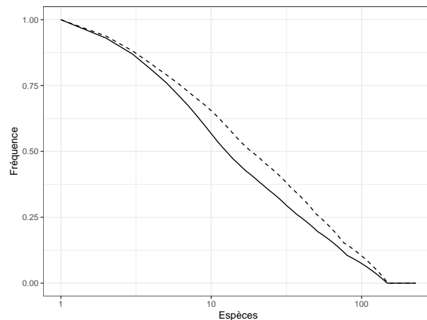
FIG. 4.6 : Profil de queue de distribution calculé pour les deux parcelles de Paracou (Parcelle 6 : trait plein et Parcelle 18 : trait pointillé). En abscisse : rang de l'espèce dans le classement de la plus fréquente à la plus rare ; en ordonnée : probabilité qu'un individu de la communauté appartienne à une espèce plus rare.
