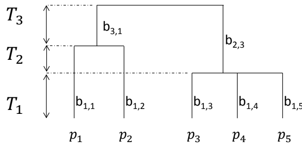
FIG. 6.1 : Arbre phylogénétique ou fonctionnel hypothétique. 5 espèces sont présentes ( S = 5 ), leurs probabilités notées p_1 à p_5 . Les noms des branches sont affichés.
