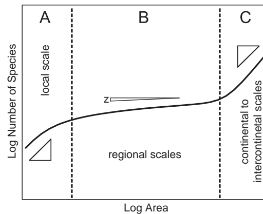
FIG. 22.6 : Relation aire-espèce triphasique [Grilli2012]. Zone B : relation d'Arrhenius.
