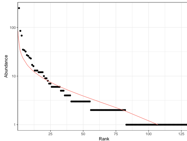
FIG. 3.1 : Echantillon de 1000 individus tiré dans une communauté log-normale.
