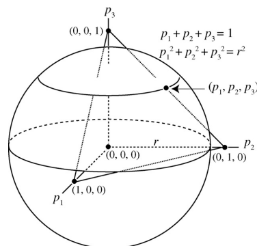
FIG. 9.5 : Représentation d'une communauté dans un espace multidimensionnel dont chaque axe correspond à une espèce. La communauté est composée de trois espèces. Le point représentant la communauté se trouve sur la sphère de rayon r = \sqrt{\sum_s p_s^2} . Le plan (qui est en réalité un hyperplan de dimension S - 1 ) d'équation \sum_s p_s = 1 est représenté par un triangle.
