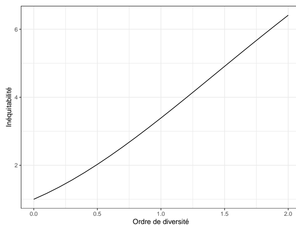
FIG. 5.2 : Profil d'inéquitabilité de BCI : L'inéquitabilité augmente quand on néglige de plus en plus les espèces rares. Pour q=2 , la forêt de BCI est aussi inéquitable qu'une communauté de 6 espèces dans laquelle une seule serait représentée au-delà d'un nombre négligeable d'individus.
