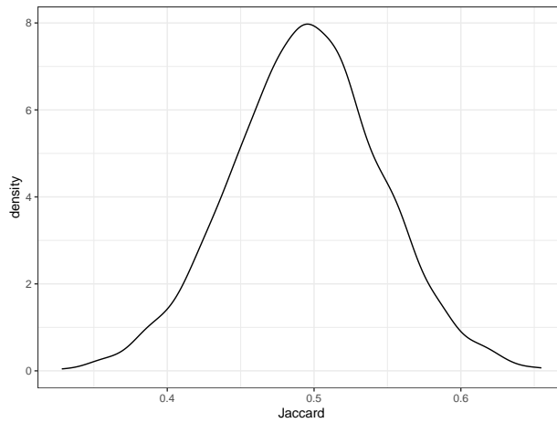
FIG. 11.1 : Distribution des indices de Jaccard calculés pour les 50 carrés de BCI deux à deux.
