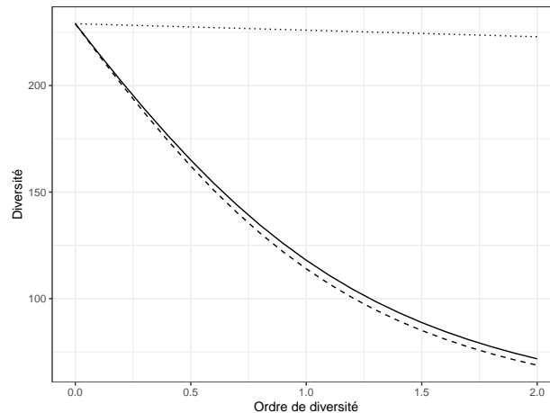
FIG. 7.6 : Profil de diversité d'abondance et fonctionnelle de Scheiner de la méta-communauté Paracou618. Pointillés longs : diversité d'abondance; pointillés courts : diversité fonctionnelle; trait plein : diversité d'abondance et fonctionnelle.
