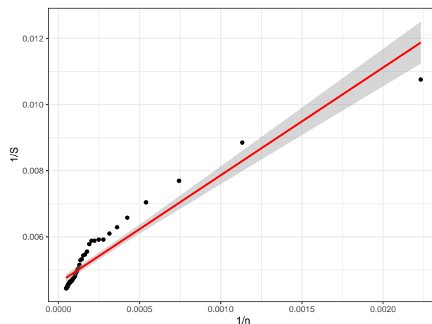
FIG. 3.6 : Ajustement du même modèle de Michaelis-Menten transformé selon Lineweaver et Burk.
