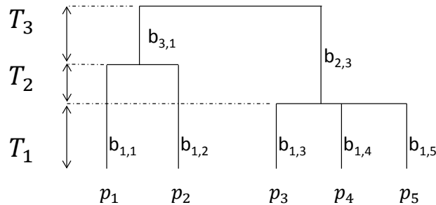
FIG. 9.4 : Arbre phylogénétique ou fonctionnel hypothétique. 5 espèces sont présentes ( S = 5 ), leurs probabilités notées p_1 à p_5 . Les noms des branches sont affichés.
