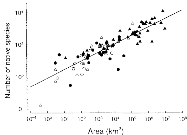
FIG. 22.1 : Logarithme du nombre d'espèces en fonction du logarithme de la surface échantillonnée. Les données sont des relevés d'espèces natives de plantes vasculaires sur 104 sites de taille variable à travers le monde. Les symboles correspondent à divers types d'habitats (îles ou continent, réserves ou non) sans intérêt ici. La valeur de z est 0,27.
