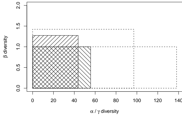
FIG. 13.1 : Représentation graphique de la diversité des deux parcelles du jeu de données Paracou618 . Les rectangles transparents représentent la diversité neutre, les rectangles hachurés la diversité phylogénétique (l'arbre est la taxonomie des espèces, q = 1 ). Dans chaque cas, le rectangle le plus large, de hauteur 1, représente la diversité gamma . Le rectangle plus haut a pour largeur et longueur les diversités \alpha et \beta . Les surfaces des deux rectangles sont identiques.
