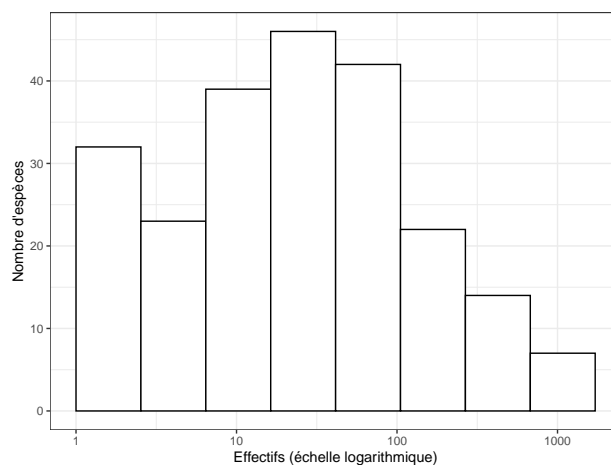
FIG. 2.2 : Histogramme des fréquences (diagramme de Preston) des arbres du dispositif de Barro Colorado Island. En abscisse : le nombre d'arbres de chaque espèce (en logarithme) ; en ordonnée : le nombre d'espèces.
