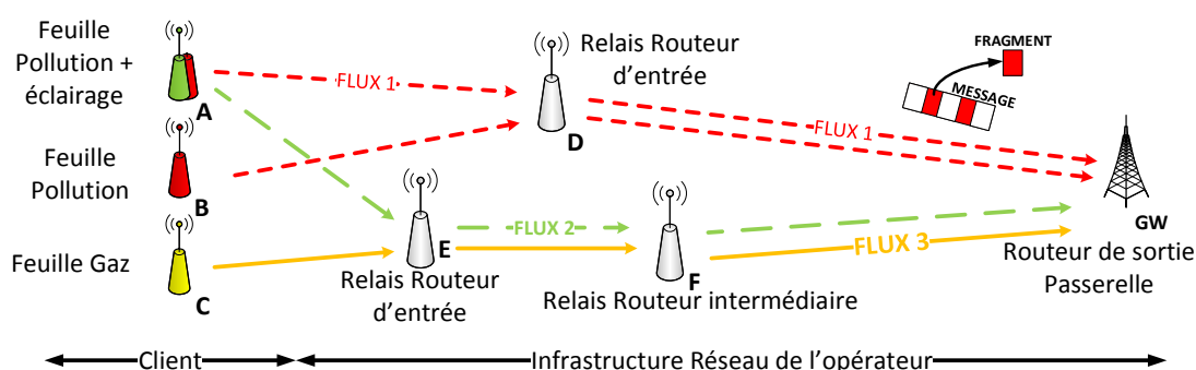
FIGURE 4.2 – Constitution du réseau de l'opérateur
