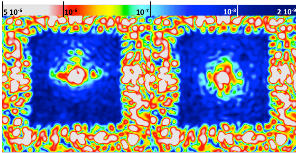
FIGURE 3.6 – Images coronagraphiques obtenues sur le THD2 avec un FQPM et une SCC en lumière monochromatique (785 nm) en minimisant l’intensité des tavelures stellaires dans tout le champ autour de l’étoile (droite) et dans la partie basse du champ uniquement (gauche). L’échelle de couleur donne le rapport de flux par rapport à l’étoile (i.e. contraste).
