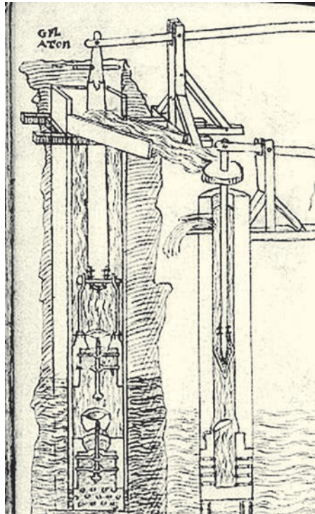
Plan de la pompe de Thon
