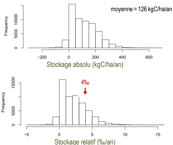
Figure 4-32. Stockage additionnel annuel moyen sur 0-30 cm avec le scénario "Insertion et allongement des CI"
