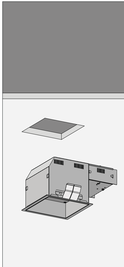
Aufbau Schematische Darstellung des Aufbaus der Down 183
