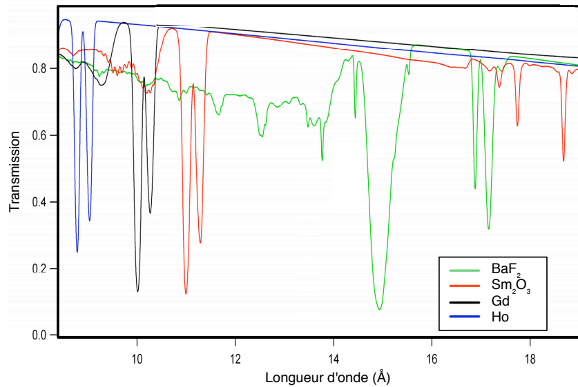
Fig. 7.1 – Prédications théoriques (SCO) pour les transmissions du fluorure de baryum, de l'oxyde de samarium, du gadolinium et du holmium. Le holmium n'a pas été retenu dans l'analyse des données expérimentales.
