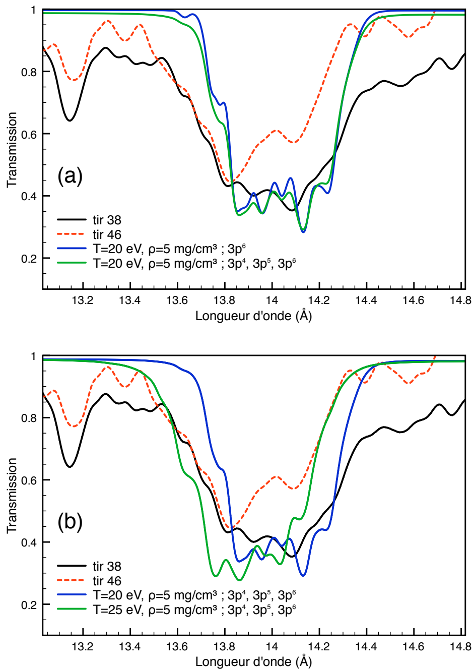
Fig. 6.14 – Transmission du nickel ( 20 \mu\text{g}/\text{cm}^2 ) pour les tirs 38 et 46 comparés aux calculs HULLAC pour les seules transitions 2p - 3d . (a) Calculs à T = 20 eV et \rho = 5 mg/cm 3 , avec une sous-couche 3p^6 fermée (bleu), ou des sous-couches 3p^6, 3p^5 et 3p^4 (vert). (b) Calculs pour les températures de 20 et 25 eV, densité de 5 mg/cm 3 . Le choix des configurations du calculs ne permettent pas de reproduire les structures 2p - 4d dont celle visible à 13.15 Å.
