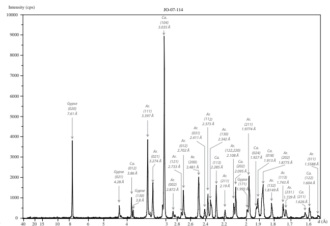
k-Diffractogramme d'échantillons de travertin provenant de la salle T1 (JO-05-34) et T7 (JO-07-114) ; (Ar: Aragonite ; Ca.: Calcite).
