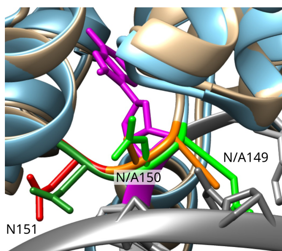
Figure 49: Vue rapprochée sur le motif NNN pour OGG1 WT (bleu) et 2NA (doré). Gris : ADN, Magenta : 8-oxoG (extrudée), Vert : Motif NNN WT, Orange : A149 et A150, Rouge : N151 (2NA). Structure WT : PDB 6w0m ; Structure 2NA : prédiction AlphaFold.
