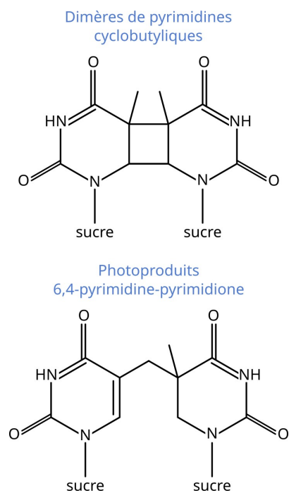
Figure 5: Dimères de pyrimidine.
