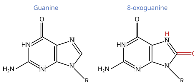
Figure 12: Différences entre la guanine (à gauche) et la 8-oxoguanine (à droite).
