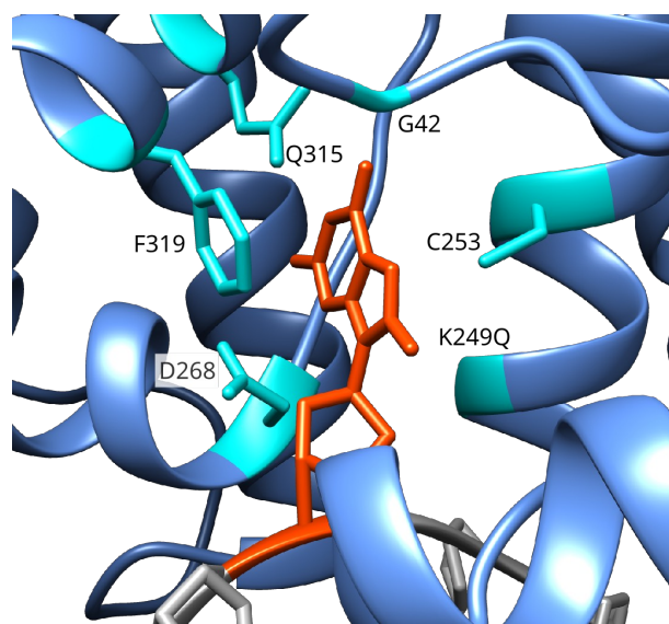
Figure 18: Structure du site actif d'OGG1 (bleu) lorsque la 8-oxoG (rouge) est extrudée. Le reste de l'ADN est en gris, les acides aminés notables et leurs chaînes latérales sont en cyan. Seule la chaîne latérale du Q249 n'est pas montrée puisqu'elle n'est pas pertinente, le résidu original étant une lysine. PDB : 1EMB.
